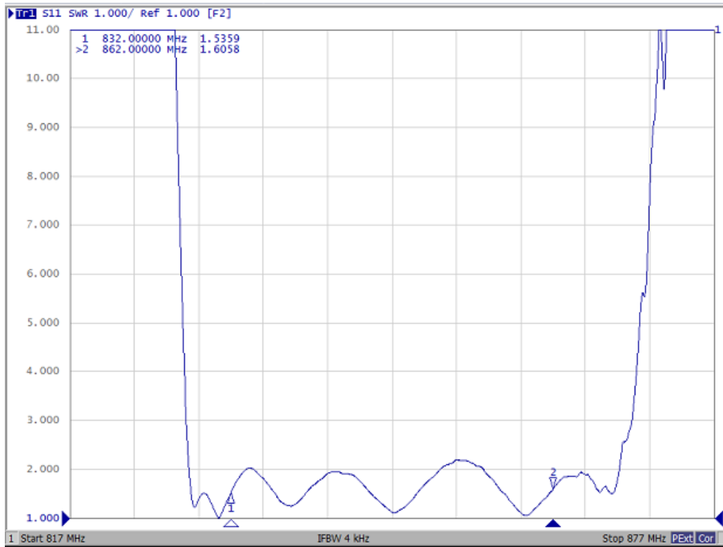
S11 VSWR
